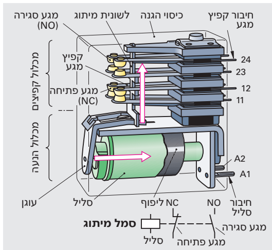
תמונה 1: ממסר
